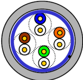
FTP
