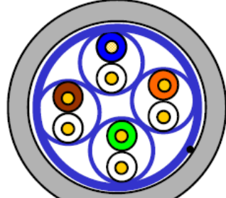
STP
